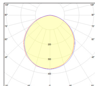
Lichtverteilungskurve WEGA CLICK ON 1.547mm
